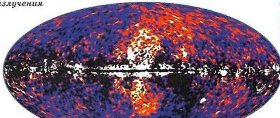
Карта распределения \gamma -излучения
