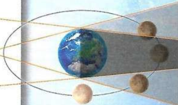
Схема лунного затмения
